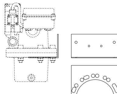
Wandhalter Wall bracket
